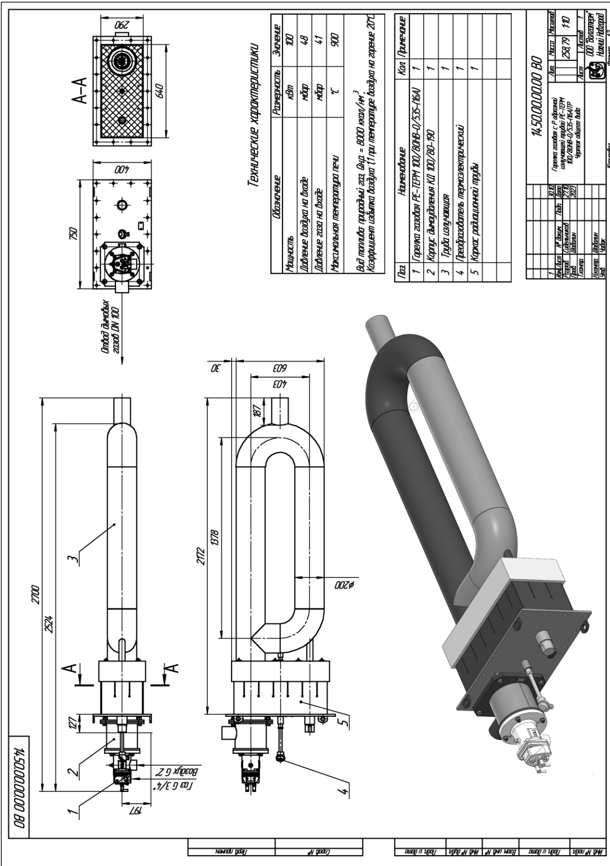
Рисунок А.1– Чертёж общего вида горелки РЕ-ТЕРМ 100/80НВ-0/535-(16А)ТР
