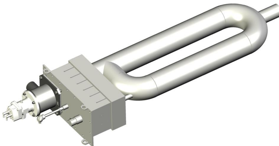
Рисунок 1 – Внешний вид горелки газовой РЕ-ТЕРМ 100/80НВ-0/535-(16А)ТР
