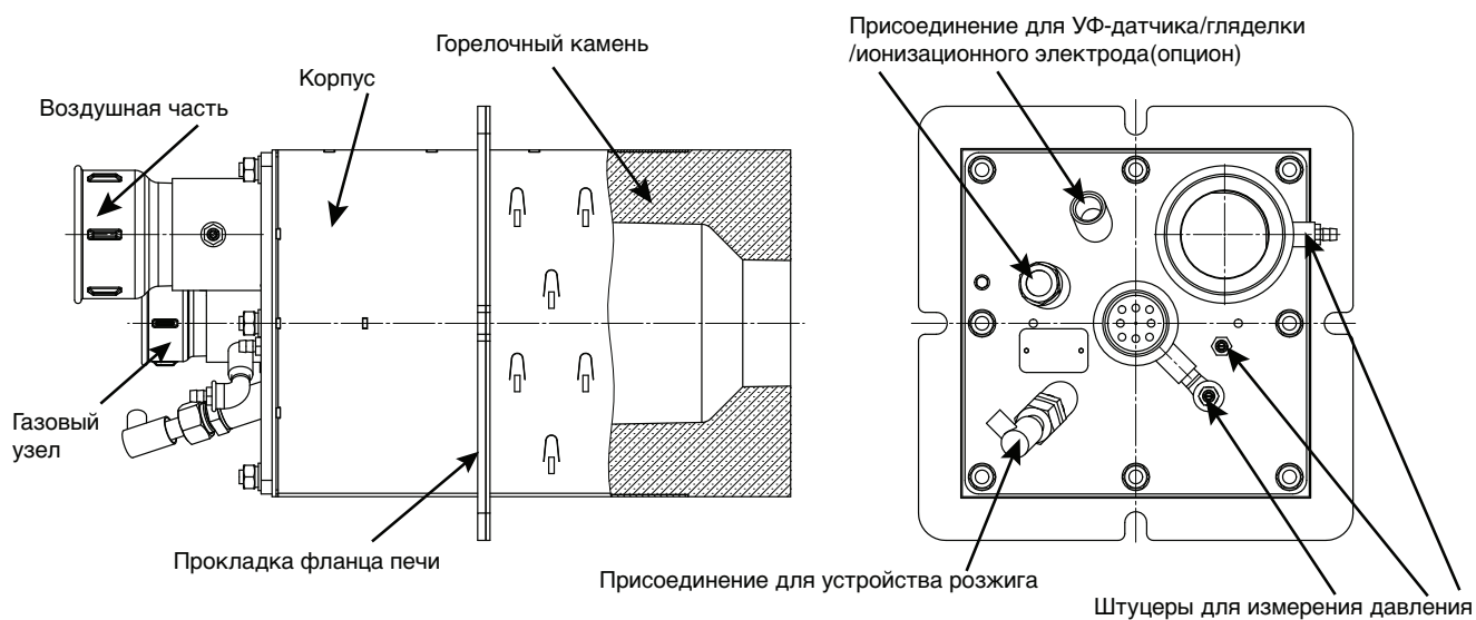
Рис. 1. Обозначение основных частей горелки ВИХРЬ с горелочным камнем.
